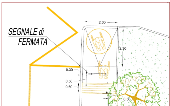
Particolare della rampa Scala 1:100
